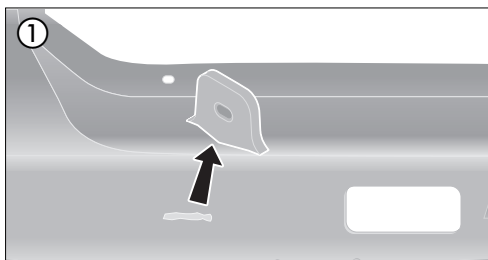
① Fixation d'une patte de guidage.
