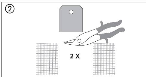
② Découper le treillis métallique en inox pour les deux côtés de la patte à la largeur de la patte. Longueur env. 60 mm, dépassant de la moitié.
