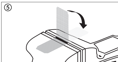
⑤ Plier séparément à 90° le treillis métallique en excès.
