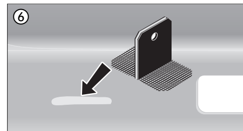
⑥ Placer la patte à l'emplacement prévu et fusionner les deux côtés dans le plastique du pare-chocs à l'aide de la buse de réparation pour automobile. La patte peut être légèrement pliée de l'autre côté afin de pouvoir travailler plus facilement sur sa base.
